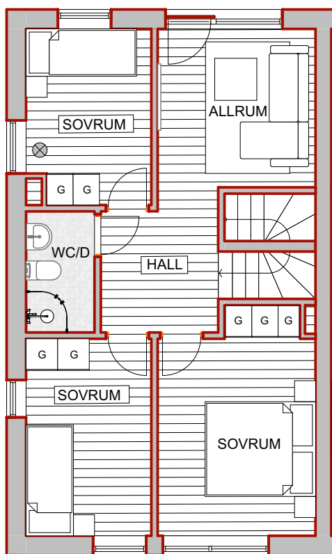
Plan 2 (6) 1:100
