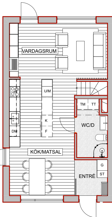
Entréplan (7) 1:100
